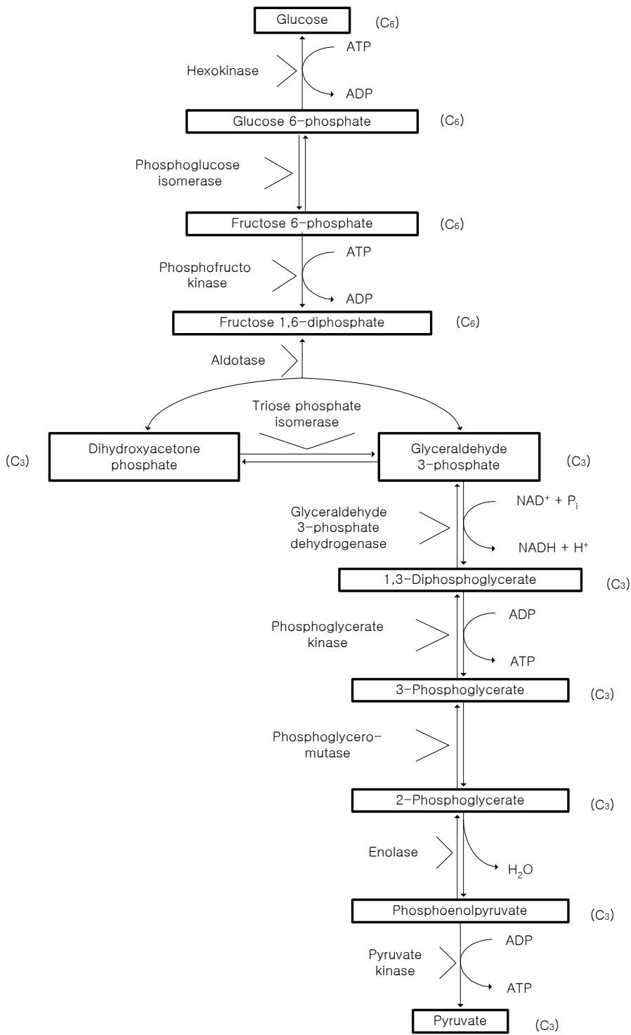
그림 4.5 해당과정(glycolytic pathway)
