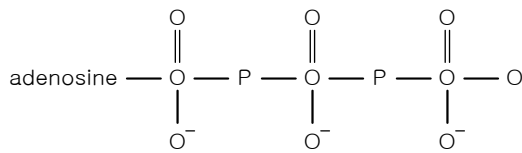
그림 4.2 ATP의 분자구조
