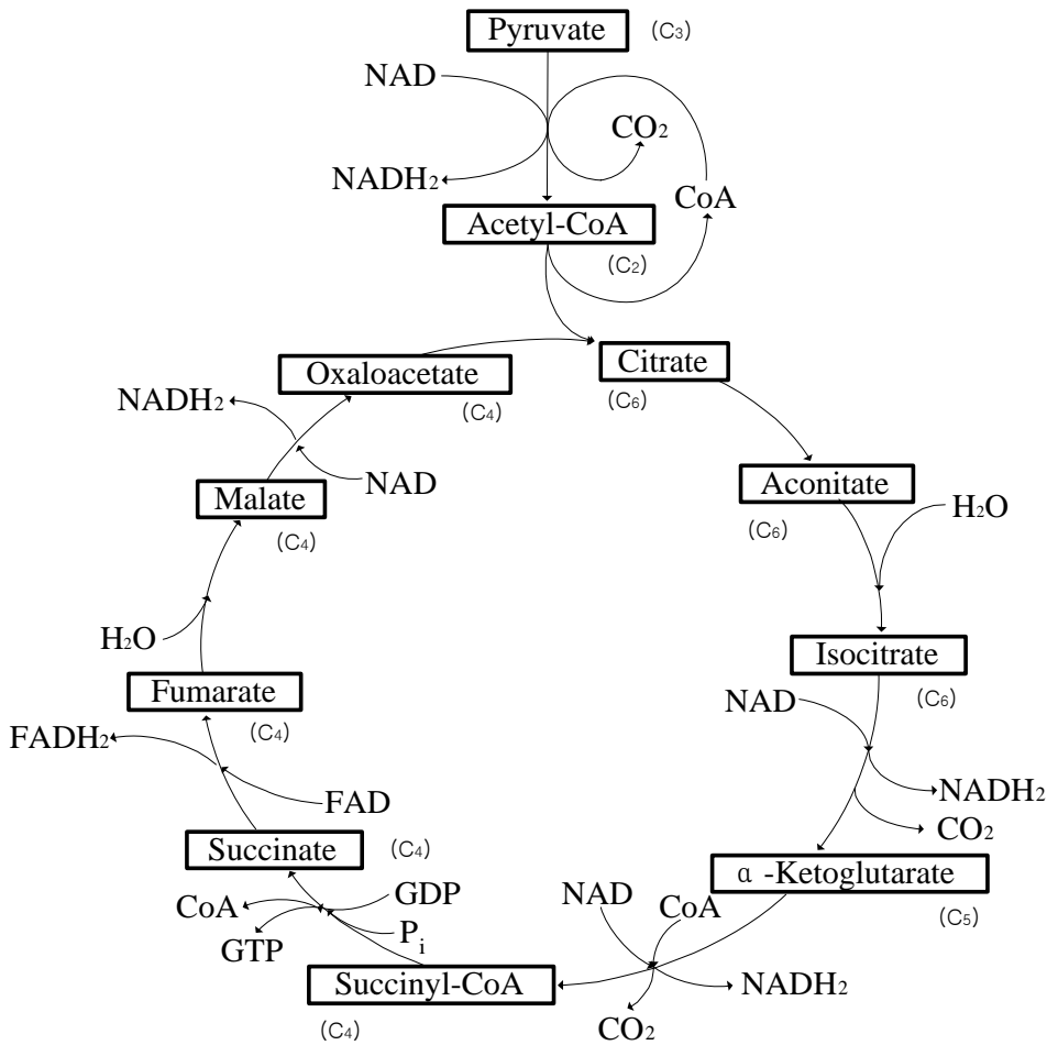
그림 4.6 TCA 회로
